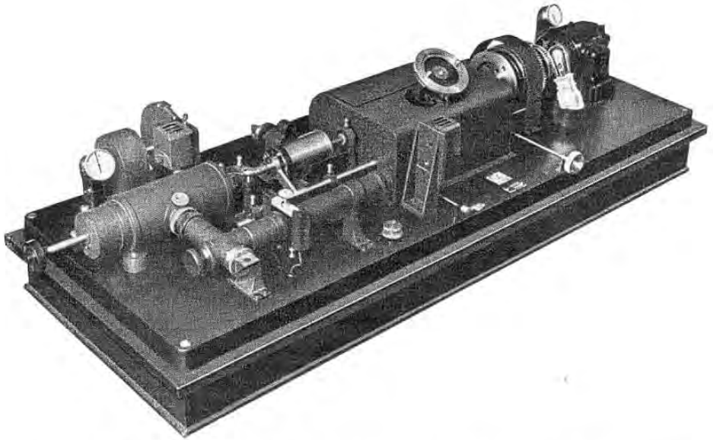
Bild 42. Faksimiletelegraph nach Telefunken-Karolus-Siemens für Duplexbetrieb mit Doppeltrommel, Ringphotozelle, Kerrlichtrelais und Gleichlaufregler. Diente für die Kurzwellenübertragungen Nauen-Rio de Janeiro, Nauen-Rom und Nauen-Moskau.
