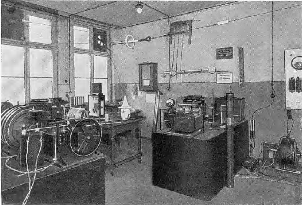
Bild 206. Raum und Einrichtung zur Senderprüfung im Telefunkenhaus, Tempelhofer Ufer 9, aus dem Jahre 1908. Xra der tönenden Funken.
