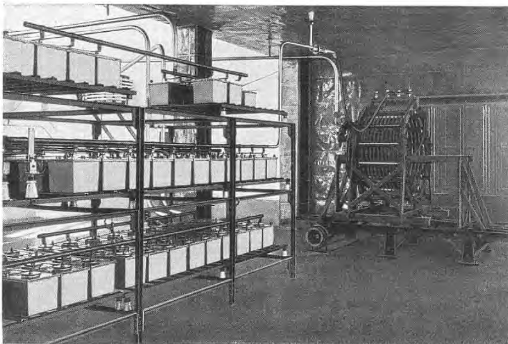
Bild 56. Batterie von Dubilier-Kondensatoren (glimmerisolierte Pakete von besonderer Fertigung), Kapazität 100000 Zentimeter pro Zelle, in der Großstation Rom. Geringer Platz- und Materialverbrauch, verschwindende Verluste, hohe Beständigkeit.
