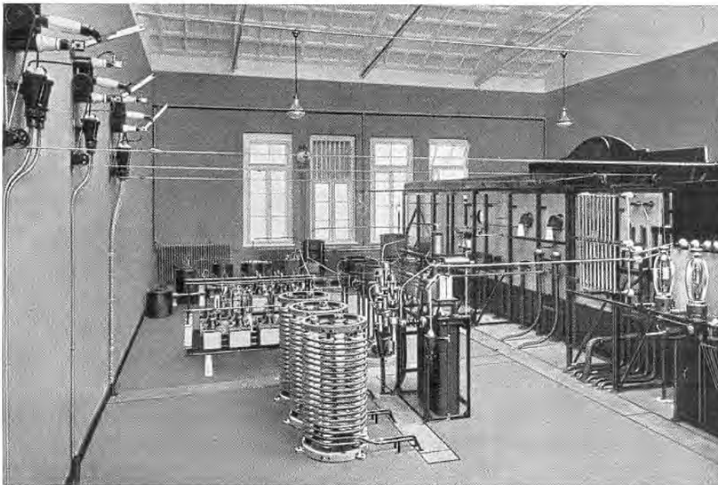
Bild 242. Blick in den Hochfrequenzraum des von Telefunken erbauten Großrundfunksenders Langenberg im Rheinland. Antennen-Telephonleistung 15 Kilowatt.
