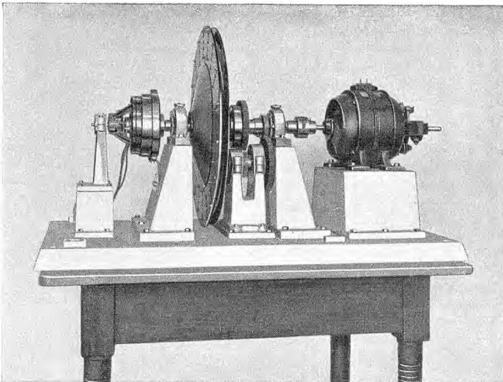
Bild 245. Fernsehermodell von Professor Dr. A. Karolus, Leipzig. Neuartiger Bildzerleger von gleicher Ausführung für Sender und Empfänger mit Antriebsmotor und Synchronhaltungsmotor.
