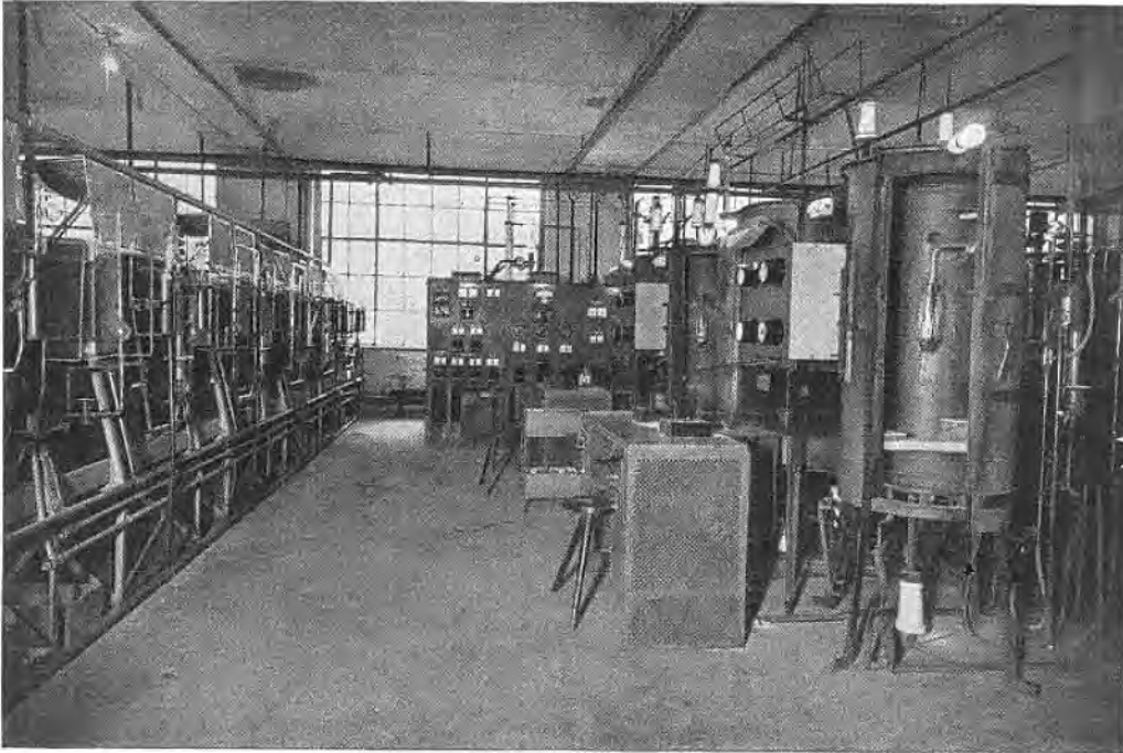
Bild 101. Die Herstellung von Telefunkenröhren im Osram-Werk A. Pumpstände für Senderöhren mit den großen hierzu notwendigen Evakuieröfen.
