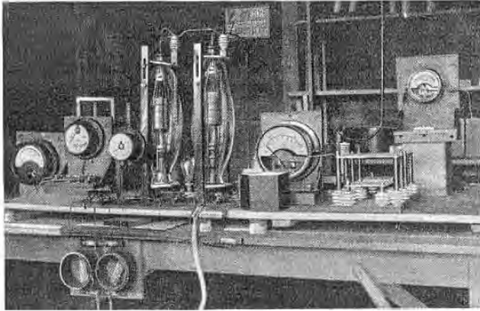
Bild 57. Ein Markstein in der Geschichte der Kurzwellentechnik: Sender pox, Nauen, mit dem der erste öffentliche Telegrammdienst nach Übersee gemacht wurde (18. Juli 1924). Wellenlänge im Anfang etwa 75 Meter, später stufenweiser Übergang zu kürzesten Wellen.
