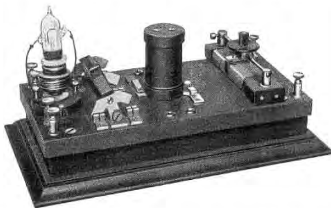
Bild 63. Erster Hochfrequenzverstärker von Otto von Bronk, 1911. Mit Glühkathodenröhre nach de Forest und Thermodetektor (Tellur/Bleiglanz).
