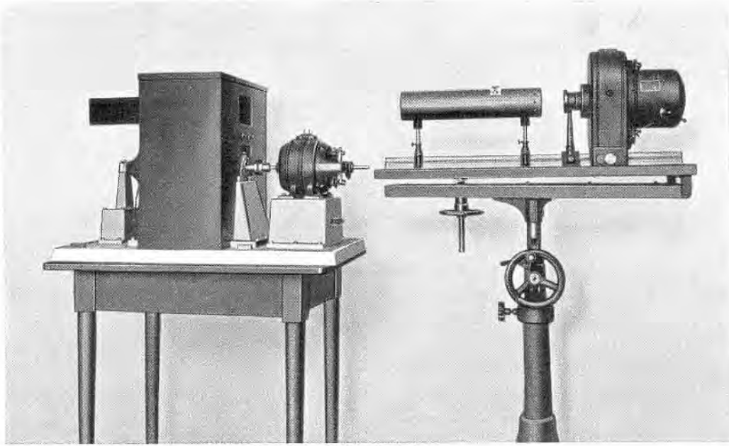
Bild 246. Fernsehmodell von Professor Dr. A. Karolus, Leipzig. Der Bildempfängerteil mit eingebauter Zerlegungseinrichtung, Bogenlampe und Kerroptik, die die Karoluszelle enthält.
