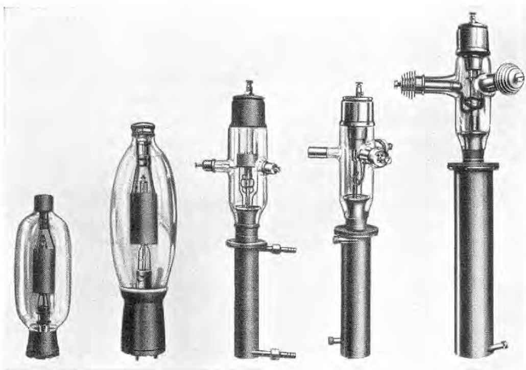
Bild 95. Entwicklungsreihe von neuzeitlichen wassergekühlten Senderöhren für Telegraphieleistungen von 10, 20 und 50 Kilowatt. Gitter- und Heizstromdurchführungen getrennt. Für kurze und lange Wellen gleichmäßig geeignet. Links daneben zum Größenvergleich die beiden luftgekühlten Senderöhren RS 47 für 1 Kilowatt und RS 53 für 2,5 Kilowatt.
