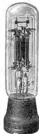
Bild 85. Erste Senderöhre Telefunks, RS 1, mit etwa 3 Watt Hochfrequenzleistung bei 440 Volt Anodenspannung. Erzeugnis der Fabrik Friedrichstraße. Modell für Schützengrabensender. Man beachte den komplizierten Bau des Elektrodensystems.
