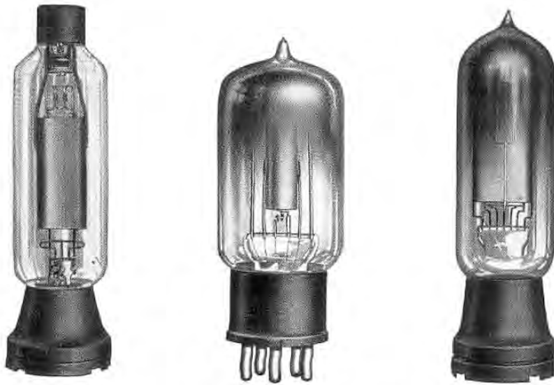
Bild 104 (links). Verstärkerröhre RV 24 mit Wolframfaden. Endstufe des Mikrophonverstärkers für Rundfunksender. Vielfach auch als Modulationsröhre für Gittergleichstromtelephonie benutzt.
