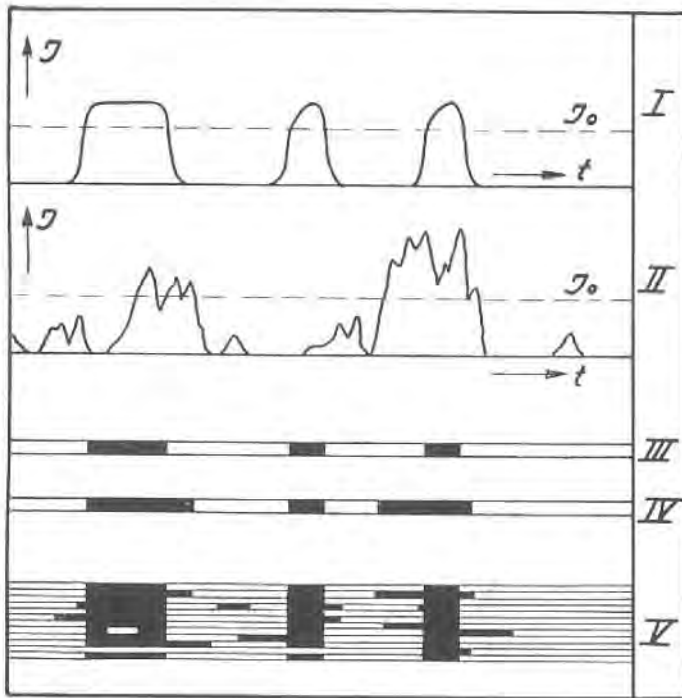
Bild 41. Darstellung der Störung von Signalphotogrammen und der Zeichenselektion durch bildliche Verschmelzung wiederholter Einzelregistrierungen.
