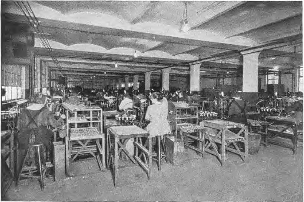
Bild 100. Die Serienfabrikation von Telefunken-Rundfunkempfangsröhren bei der Osram-Kommanditgesellschaft, Werk A, Sickingenstraße. Einer der Säle für maschinelle Einschmelzung der Elektroenträger.
