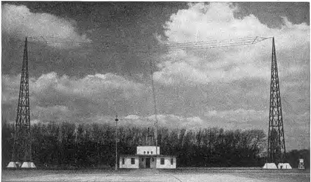
Bild 236. Flughafenstation Tempelhof-Berlin mit maximal 2 Antennenkilowatt zum telegraphischen und telephonischen Verkehr mit Flugzeugen und Flughäfen.
