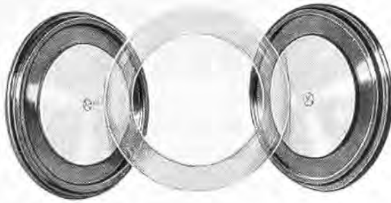
Bild 13. Ein Element der bekannten Serien-Stoßfunkenstrecke des Löschfunken senders, auseinandergenommen, in der Mitte der Glimmerring.
