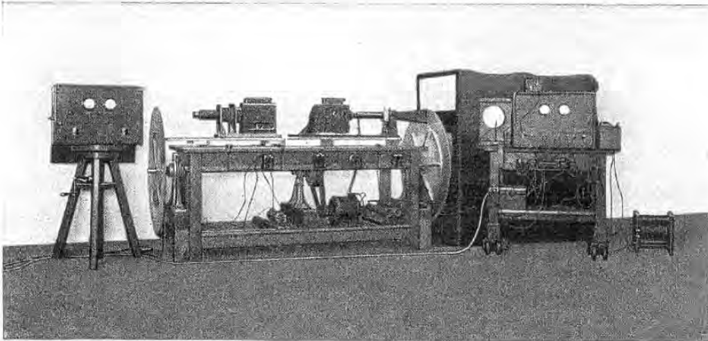
Bild 244. Modell für prinzipielle Fernsehversuche von Professor Dr. A. Karolus, Leipzig, Herbst 1924. Links Senderteil, rechts Empfängerteil. Die Nipkow'schen Bilderlegerscheiben sitzen zur Ausschaltung von Synchronismusfehlern bei diesen Voruntersuchungen noch auf gleicher Welle.
