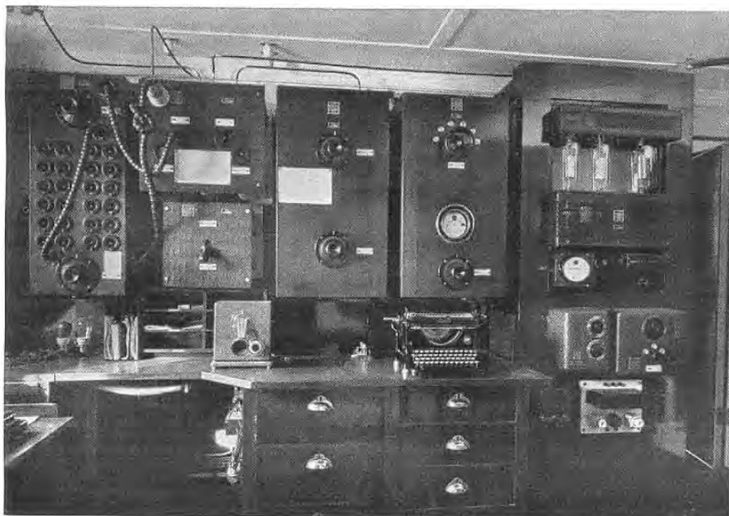
Bild 183. 1 Kilowatt-Zwischenkreisröhrensender mit Telephoniczusatz auf dem Dampfer „New York“ der Hamburg-Amerika-Linie. Wellenbereich 600 bis etwa 3000 Meter
