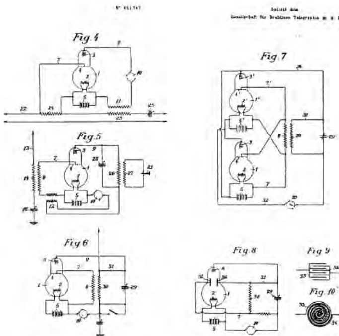
Bild 65, Figurenseite des beschlagnahmten französischen Patentes Nr. 467747 auf die Rückkopplungschaltung von Kathodenröhren nach Meißner. Umfaßt in Figuren 4 bis 7 die wesentlichsten Anordnungen für Senden, Überlagerung und Dämpfungsreduktion.
