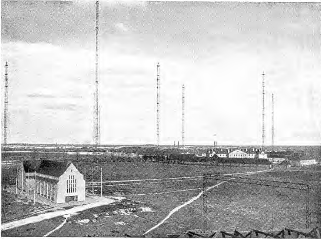
Bild 240. Teilansicht der Hauptfunkstelle Königswusterhausen. Im Vordergrunde das Senderhaus, in dem mehrere Telefunken-Großröhrensender (20 Kilowatt und 60 Kilowatt) untergebracht sind. Zwischen 13 Masten hängen 18 Antennen.
