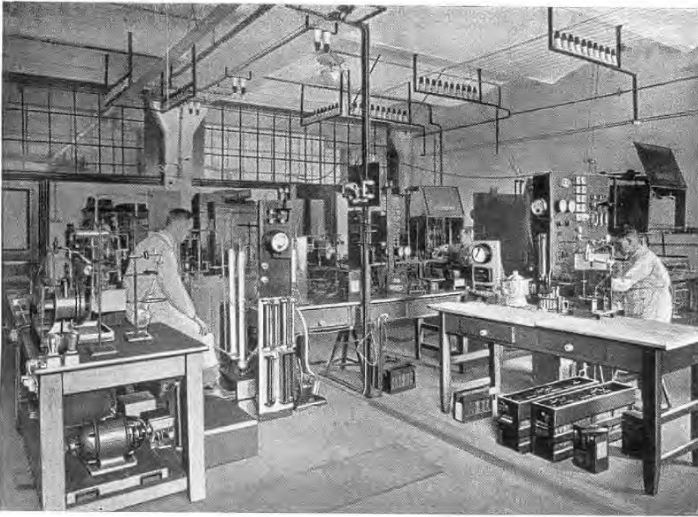
Bild 18. Telefunken-Röhrenlaboratorium Sickingenstraße: Raum für Vakuum- und Glühfädenarbeiten. in der Mitte eine Reinigungsanlage für Argongas zu Versuchen mit Glühlichtverstärkern nach Schröter-Marx (1921). (Siehe auch die Ausführungen von Hans Rukop.)
