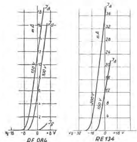
Bild 73. Kennlinien der Rundfunkempfangsröhren RE 084 und RE 134. Große Steilheit, 2 Milliampere/Volt, Durchgriff 6 0 / 10 und 10 0 / 10 .
