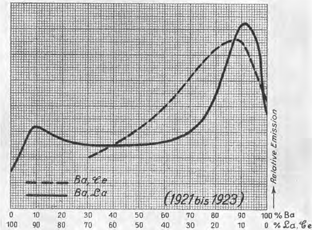
Bild 71. Aus der Entwicklung der Telefunkeröhren mit Oxydkathode: Diagramme der relativen Emission bei verschiedenen Mischungsverhältnissen zweier Oxyde (1921). Die Kurve Bariumoxyd-Lanthanoxyd zeigt zwei Maxima, denen solche der Lebensdauer entsprechen (Seite 132/133).
