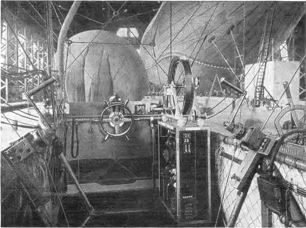
Bild 234. Erste Luftschiff-Sende- und -Empfangsanlage nach dem Löschfunkensystem, eingebaut in die Gondel eines unstarren Lenkballons (1910).
