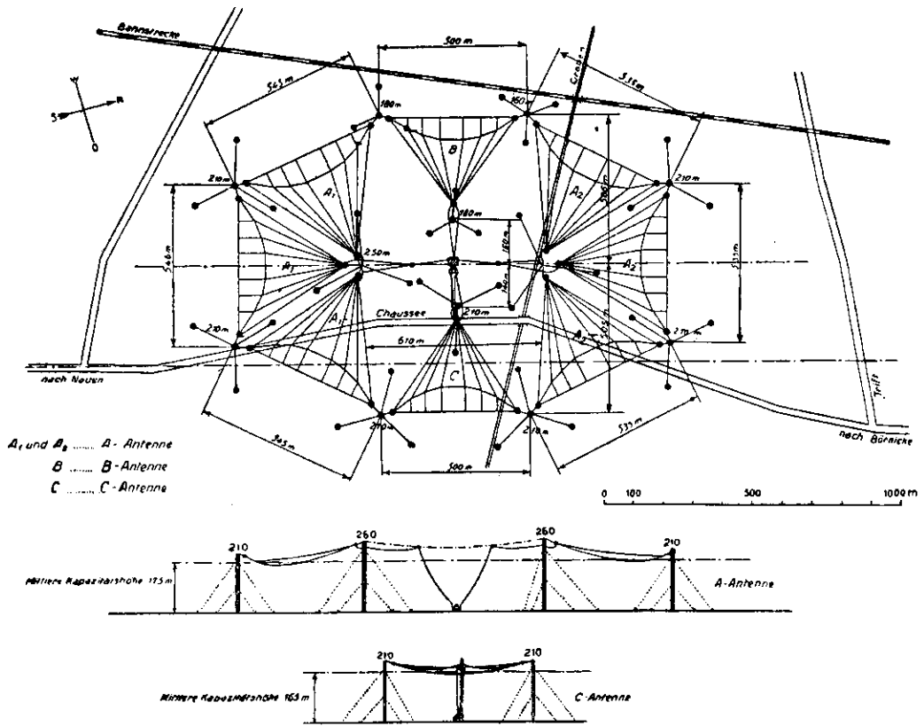
Bild 166. Die Nauener-Antennen von 1924: Vieleckform. Die Amerika-Antenne besteht aus 2 einzeln oder gemeinschaftlich benutzbaren Gruppen A_1 und A_2 , diese wiederum aus je 3 Sektoren. Heute tragen die 12 Masten (Höhe bis 260 Meter) außer den hier gezeigten Flächenantennen noch 4 mehrdrähtige T-Antennen
