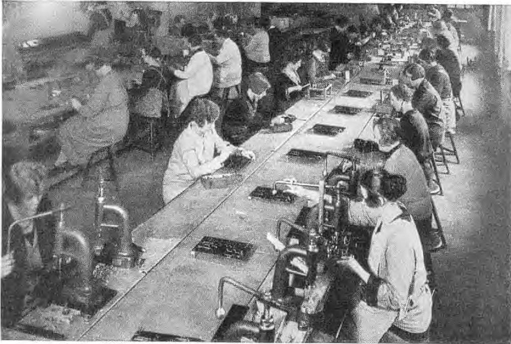
Bild 125. Aus den Funkwerkstätten bei der A. E. G. Montage des Rundfunkempfängers „Telefunken 4“ auf einem modernen Wandertisch.
