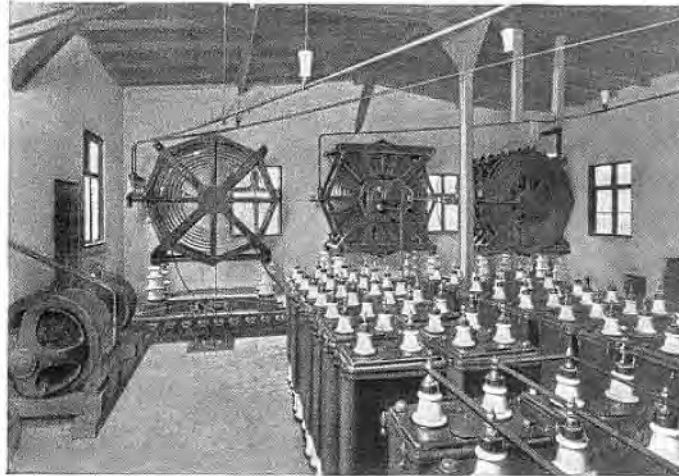
Bild 158. Vom Ausbau der Großstation Nauen: Behelfsmäßige Maschinensenderanlage aus den Jahren 1914/1915. Kondensatoren und Abstimmspulen.
