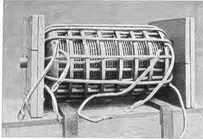
Bild 51. Frequenzwandler alter Konstruktion eines Hochfrequenzmaschinen-senders für etwa 150 Kilowatt bei 12 bis 15 Kilometer Wellenlänge. Viel Eisen, geringe Materialausnutzung, große Verluste.
