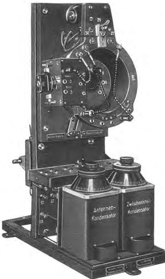
Bild 14. Detektor - Zwischenkreisempfänger E 5 für alle Wellenlängen. Bildet noch heute die Gegenanlage zum tönenden Lös-funkensender.
