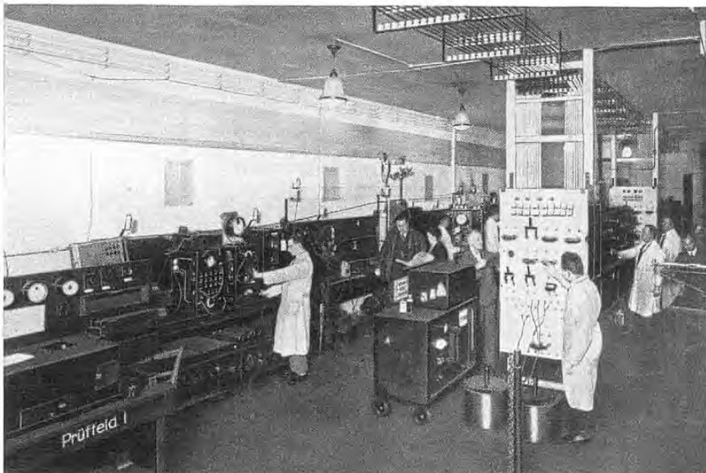
Bild 112. Das zur Telefunken-Versuchswerkstatt I gehörige Senderprüffeld. Man sieht hier die Prüfung von Zwischenkreisröhrendendern.
