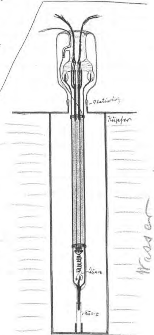
Bild 87. Erster Entwurf einer Wasserkühl-Senderöhre für 5 Kilowatt. Handzeichnung von Hans Rukop.
