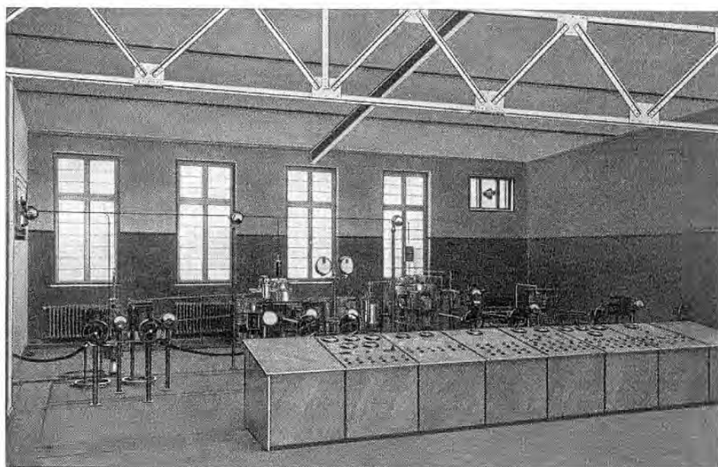
Bild 31. Hochfrequenzraum des neuen Deutschland-Rundfunksenders bei Königswusterhausen, Welle 1250 Meter, Antennen-Telephonieleistung 35 Kilowatt. In der letzten Stufe 6 Wasserkühlröhren der 20 Kilowatt-Type. Vorn das Bedienungspult mit der automatischen Druckknopfsteuerung.
