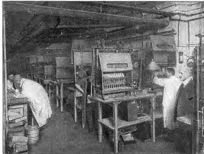
Bild 21. Aus der Zeit der Telefunken-Röhrenfabrik Friedrichstraße, 1917 bis 1920; Blick in den Pumpenraum mit 32 Evakuieröfen, in denen täglich bis zu 2000 Röhren verarbeitet wurden. Ganz rechts A. Bardehle, links K. Froberg und A. Kühne. (Siehe H. Rukop, Die Telefunkenröhren und ihre Geschichte.)
