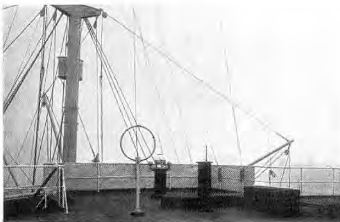
Bild 186. Rahmen des Funkpeilers auf dem Brückenhausdeck des Dampfers „Cap Arcona“.
