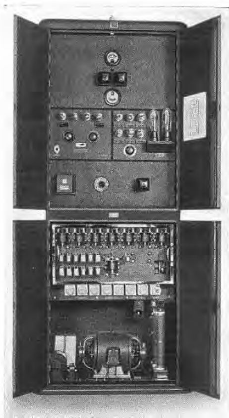
Bild 33. Neue Röhrenstation für Elektrizitätswerks-Hochfrequenztelephonie längs Starkstromleitungen. Type Station 259 EW mit selbsttätiger Wellenum-schaltung und Ladung einer Zentralbatterie, für Betrieb über gewöhnliche Postleitungen und Selbst-anschlußämter.
