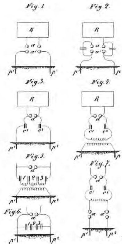
Bild 61. Figurenseite des Patentes Nr. 115081 von Ferdinand Braun über Telegraphie ohne fortlaufende Leitung. Hier handelt es sich jedoch um die Ausbreitung der Hochfrequenzwellen nicht durch den Raum, sondern in einer leitenden Oberfläche.
